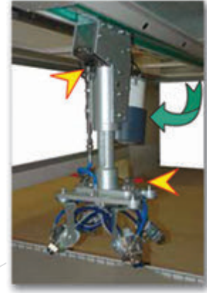
Sprey kafasını çabuk değiştirmek için "Hızlı Bağlantı" sistemi
